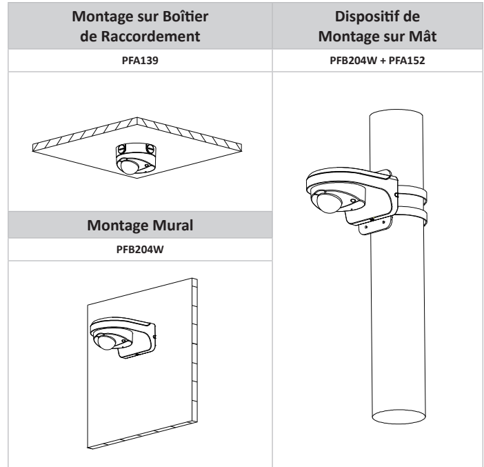
PFA152 Dispositif de Montage sur Mât
